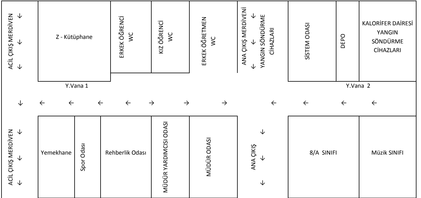
LALAPAŞA CUMHURİYET ORTAOKULU 1. KAT PLANI
